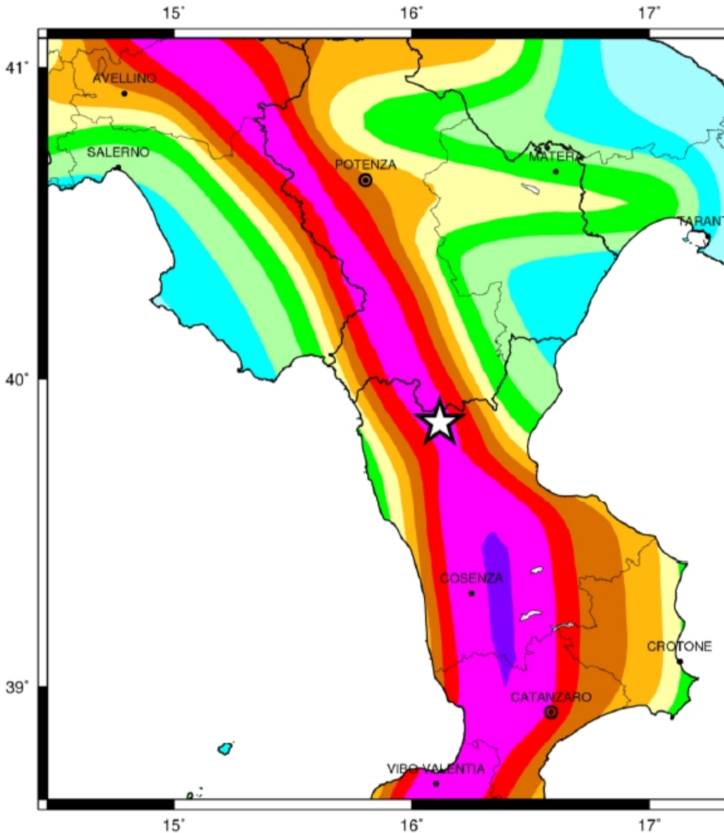
Pericolosità Sismica espressa in accelerazione massima del suolo con probab di eccedenza del 10% in 50 anni riferita a suoli rigidi
